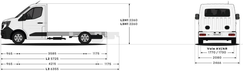
sasiu cabina (mm)
