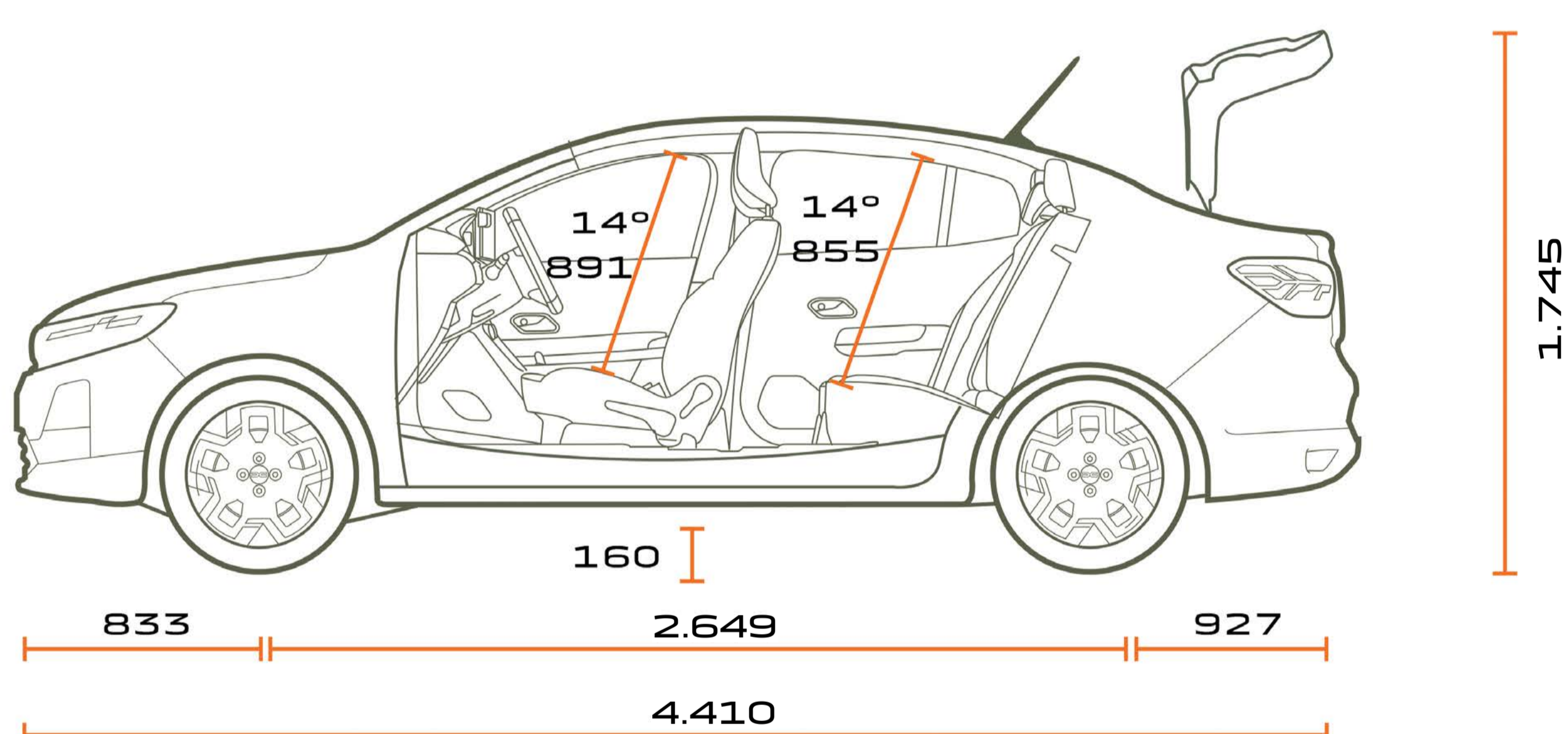
VEDERE LATERALĂ
