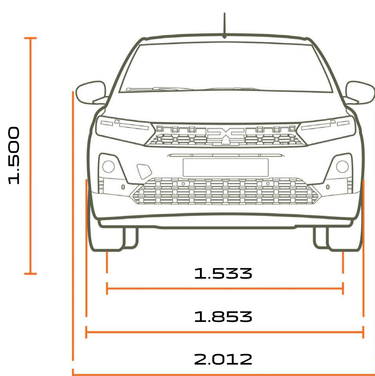
VEDERE FRONTALĂ
