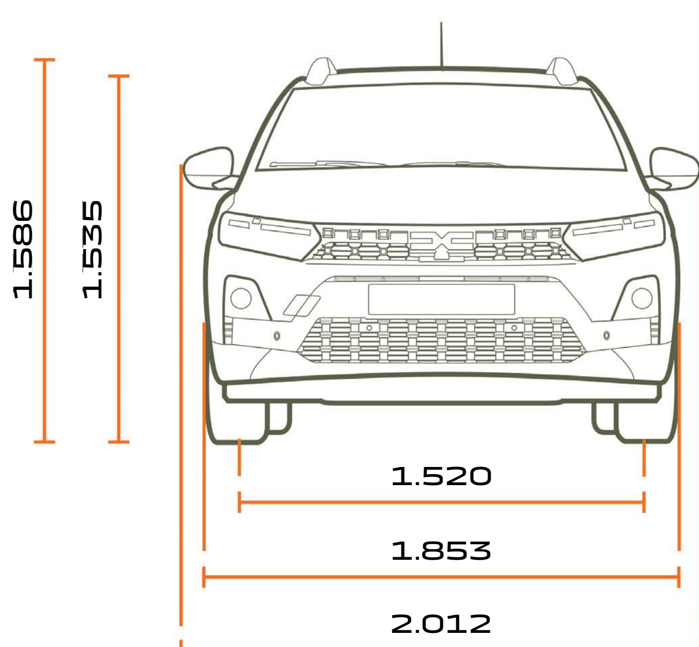
VEDERE FRONTALĂ
