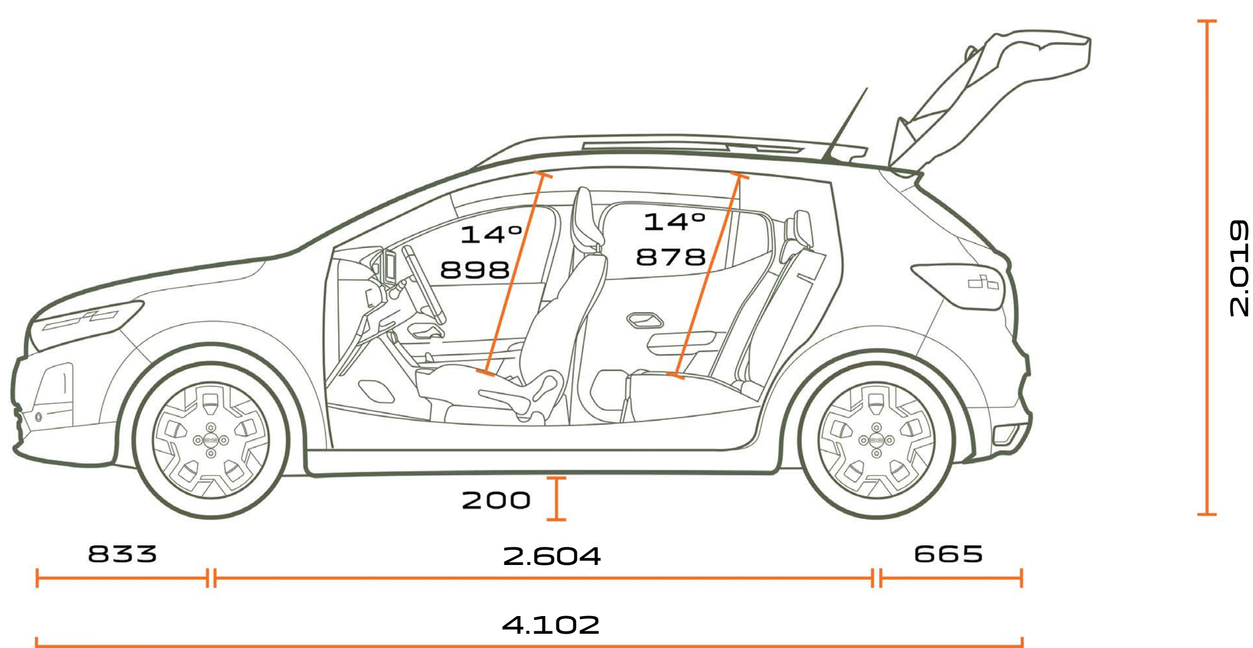
VEDERE LATERALĂ
