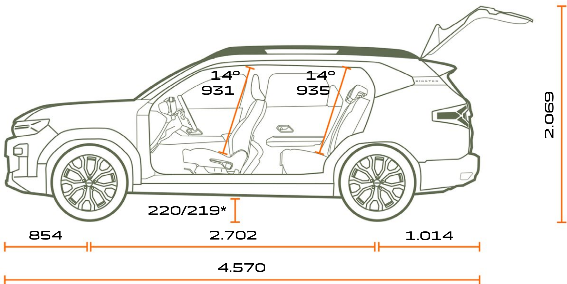
VEDERE LATERALĂ
