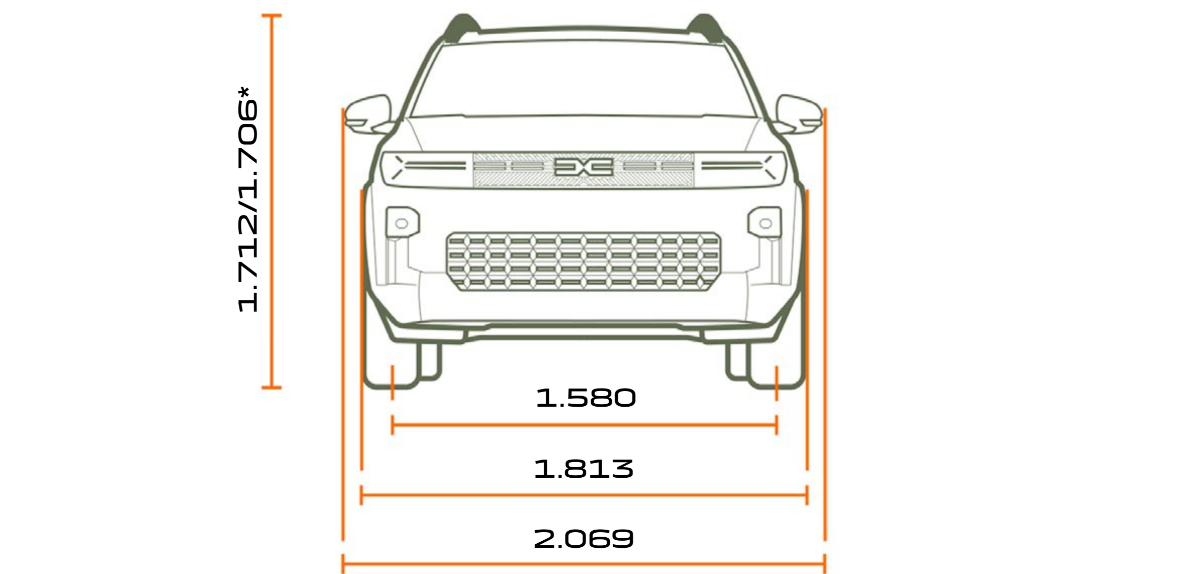
VEDERE FRONTALĂ
